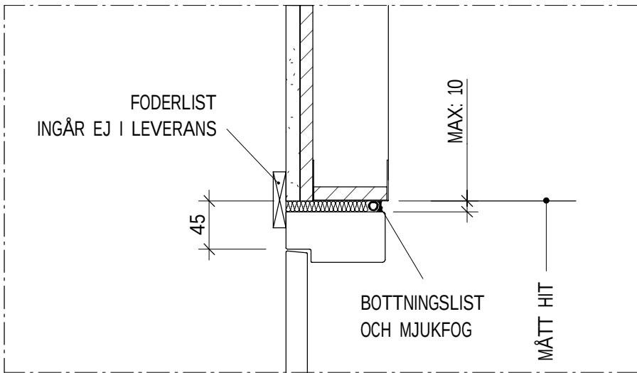
DET.A 1 : 5
