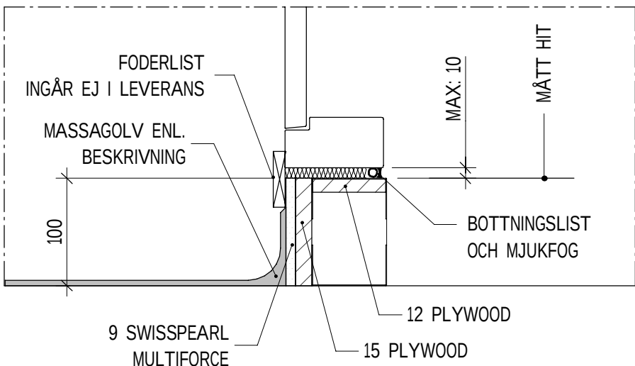
DET.C 1 : 5
